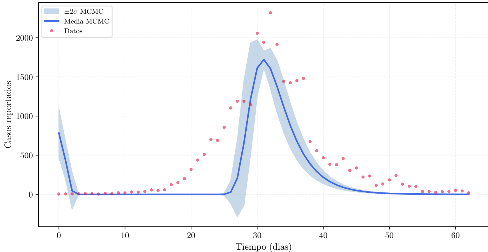
Incidencia - Modelo SEIR con incertidumbre
